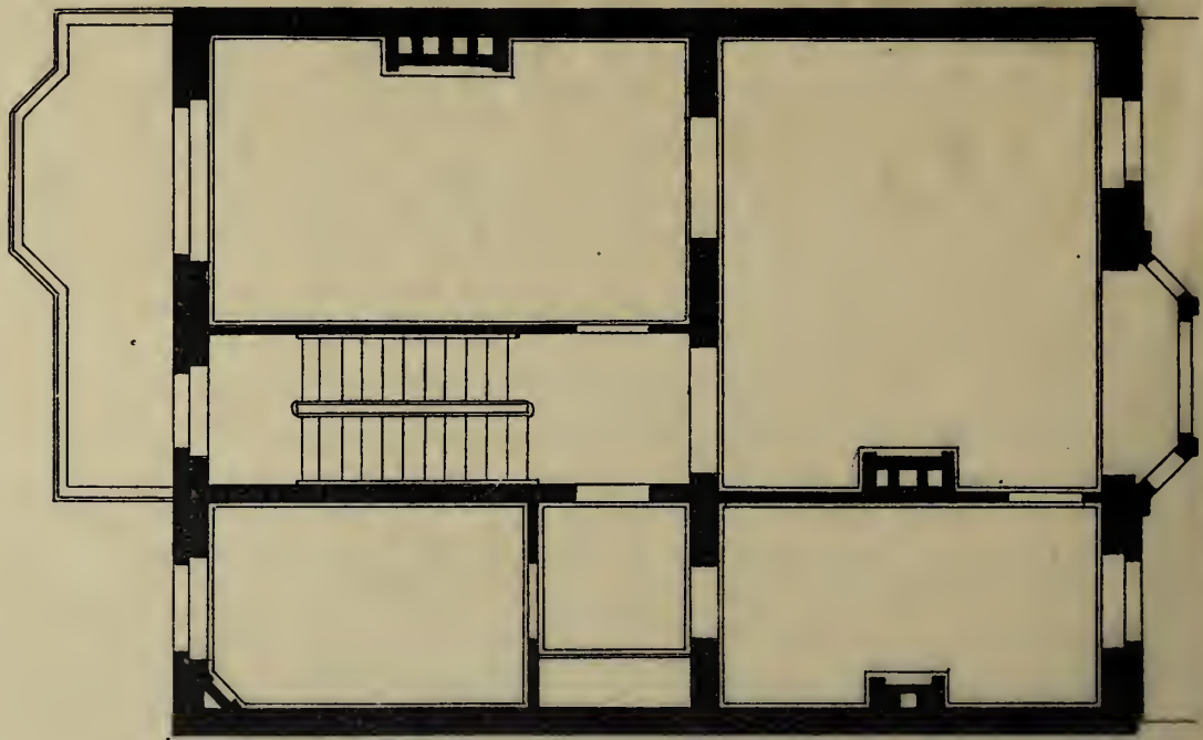
PLAN DU 1ER ETAGE
